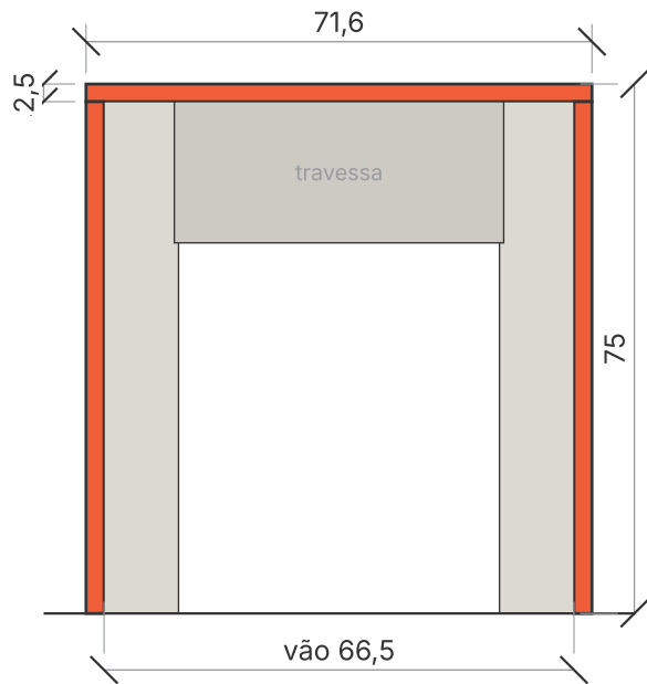
03 Mesa · elevação frontal
