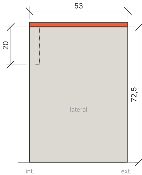
04 Mesa · lateral (VG)
