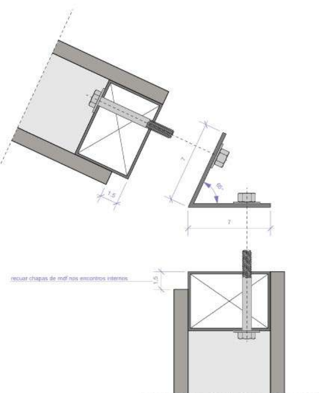
CANTONEIRAS 65° - PLANTA esc. 1:2
