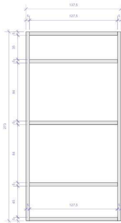
CORTE LONGITUDINAL (sem fechamento de MDF) esc. 1:20
