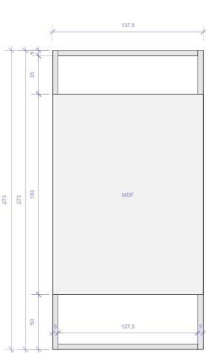
VISTA FRONTAL (com fechamento de MDF) esc. 1:20
