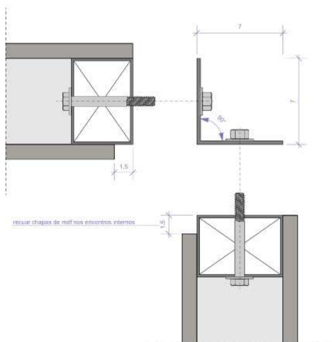
CANTONEIRAS 90° - PLANTA esc. 1:2
