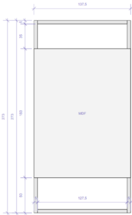
VISTA FRONTAL (com fechamento de MDF) esc. 1:20
