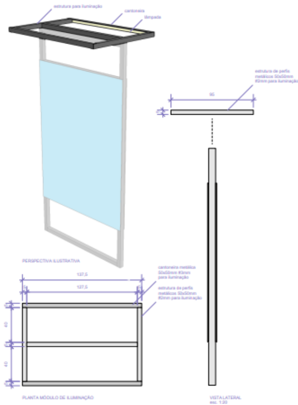
PLANTA MÓDULO DE ILUMINAÇÃO
