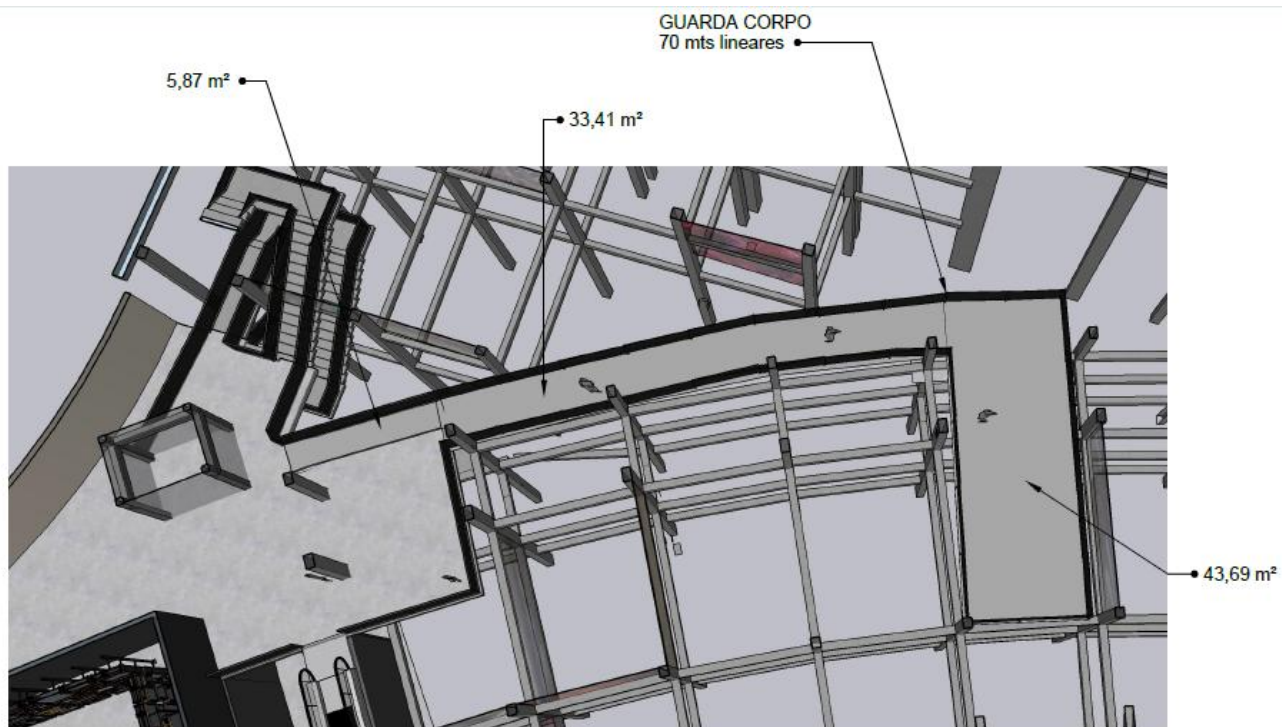
VISTA SUPERIOR - PASSARELA EXALTAÇÃO SEM ESC.
