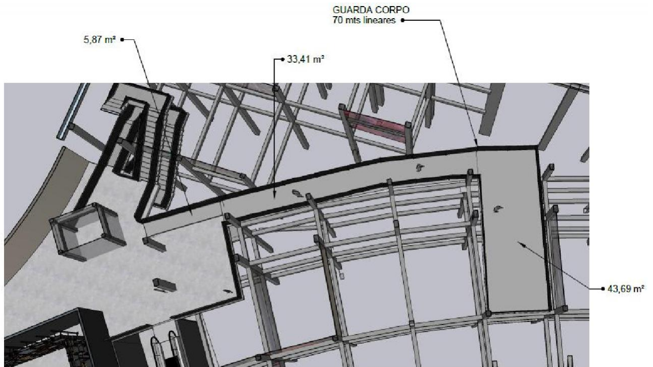
VISTA SUPERIOR - PASSARELA EXALTAÇÃO SEM ESC.
